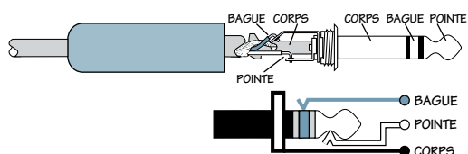
Figure B : Connecteur Jack 6,35 mm symétrique
