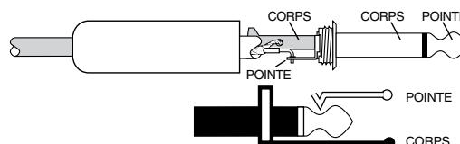
Figure C : Connecteur Jack 6,35 mm asymétrique
