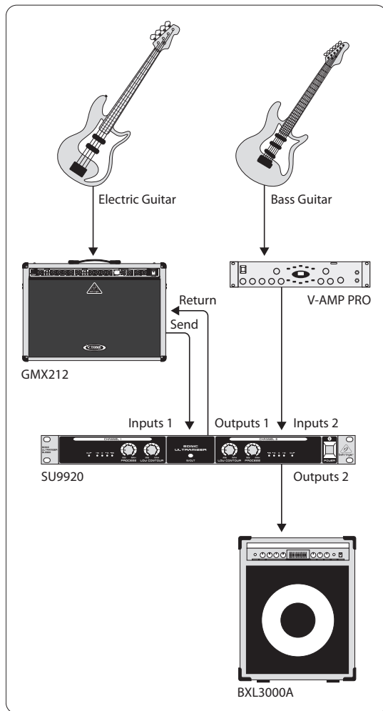
Afb. 3.3: De SU9920 bij de inzet met gitaarversterkers.
