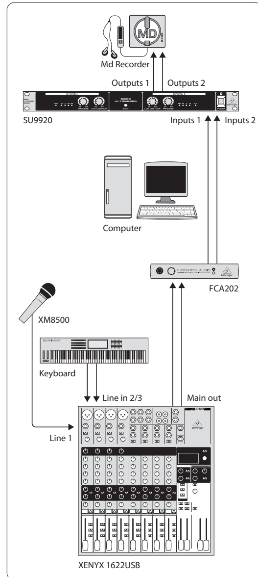
Afb. 3.2: De SU9920 in de studio
