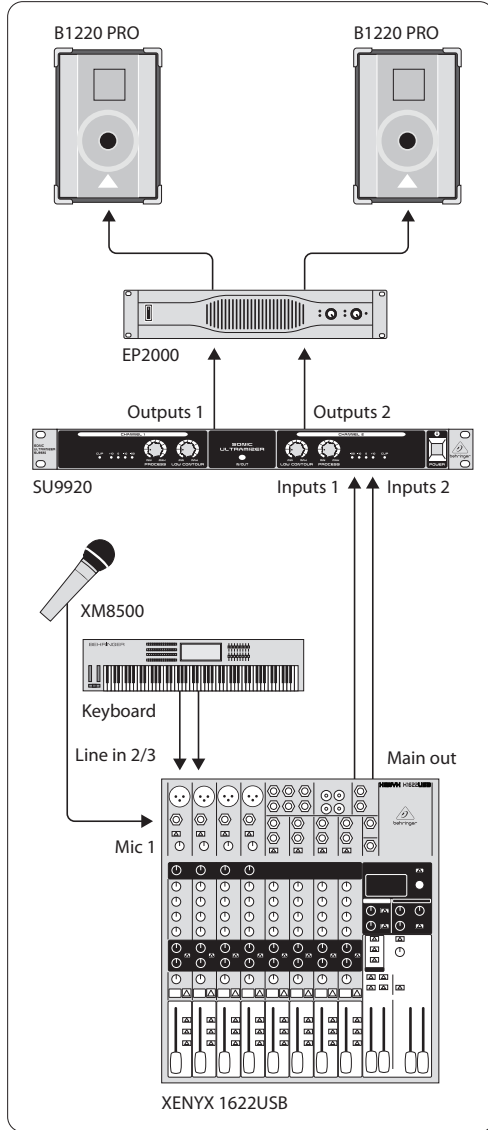
Afb. 3.1: Inzet van de SU9920 met geluidsinstallaties
