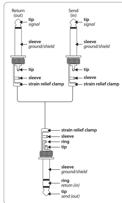
Afb. 4.4: Insert-kabel met twee monoklinker- en een stereoklinkerstekker
