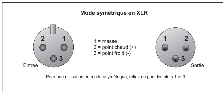
Fig. 4.1 : Les différents types de câblage
