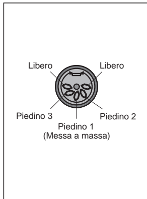
Connettore MIDI (2 piedini non sono occupati)
