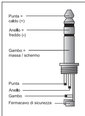
Connettore 6,3 mm, 3,5 mm & TT (il piedino 3 non deve essere necessariamente occupato)
