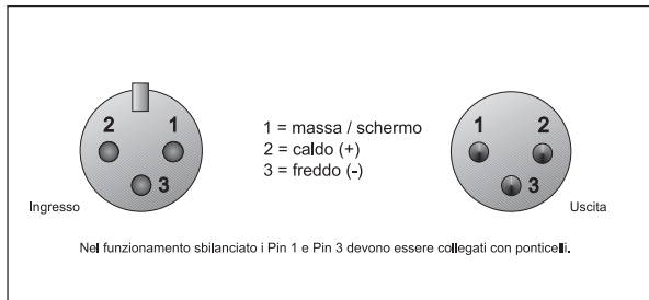
Connettore XLR (i piedini sono indicati sul connettore)
