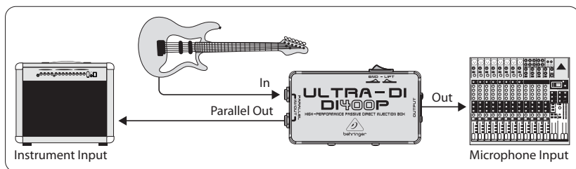
Rys. 2: Gitara → DI-Box → Wzmacniacz gitary / stół mikserski
