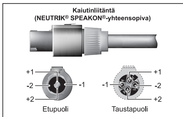
Kuva 3.1: Kaiutinliitännät (Neutrik® Speakon®-yhteensopiva)
