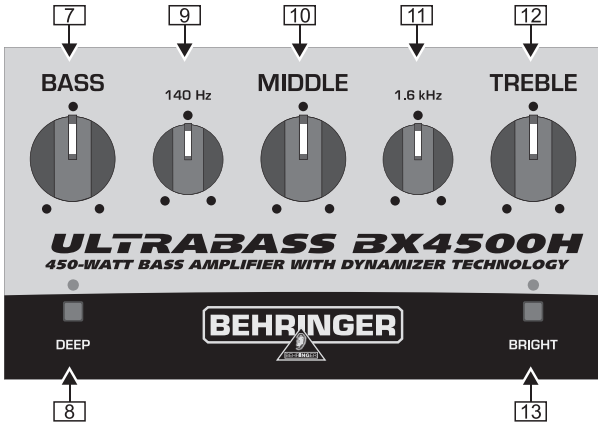
Kuva 2.2: Etupuolen käyttöelementit (Poikkileikkaus 2)
