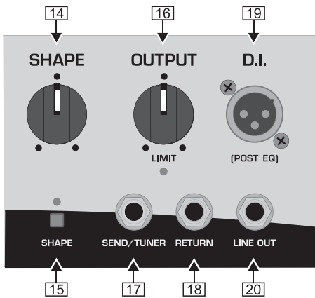
Kuva 2.3: Etupuolen käyttöelementit (Poikkileikkaus 3)
