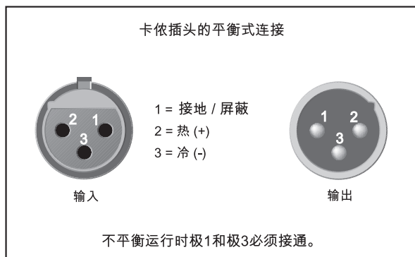
图 7.3: 6.3 卡侬接插件
