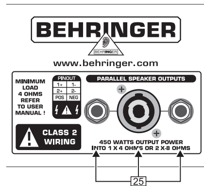
图 2.5: BX4500H 的背板 (第 2 区段)
