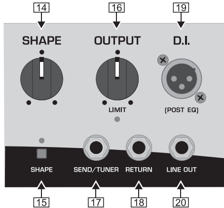
图 2.3: BX4500H 的面板 (第 3 区段)
