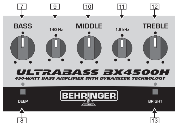
图 2.2: BX4500H 的面板 (第 2 区段)
