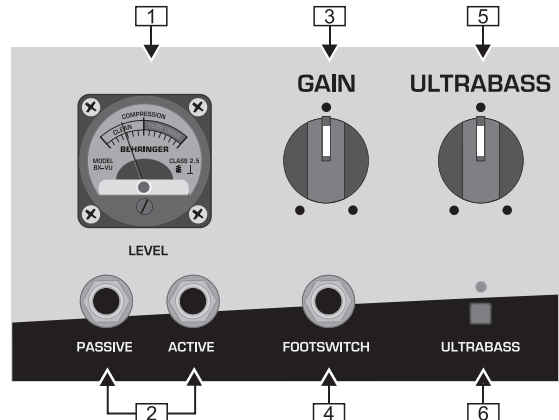
图 2.1: BX4500H 的面板 (第 1 区段)
