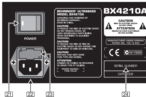
Εικ. 2.4: Πίσω πλευρά του BX4210A/BX4210 (τμήμα 1)
