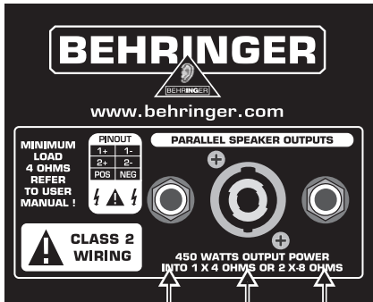
Εικ. 2.5: Πίσω πλευρά του BX4210A/BX4210 (τμήμα 2)
