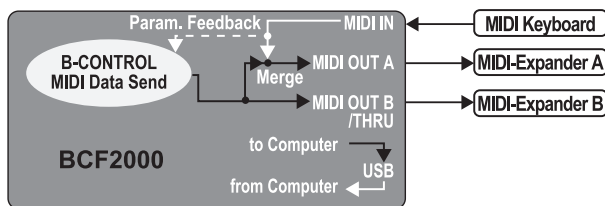
Bild 4.8: Routing och användning i Stand Alone-mode 3
