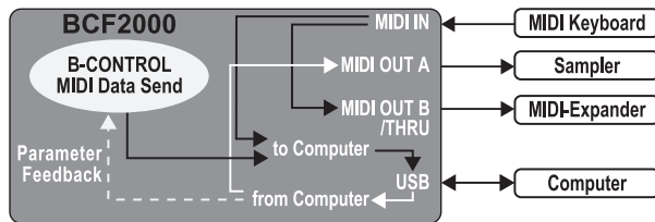
Bild 4.2: Routing och användning i USB 2
