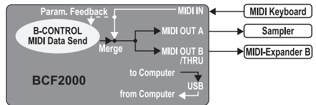
Bild 4.7: Routing och användning i Stand Alone-Mode 2
