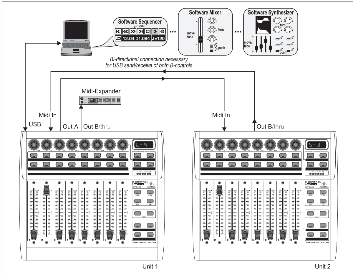
Bild 4.4: USB-Mode 4 (Expanded)
