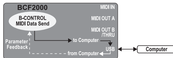
Bild 4.1: Routing och användning i USB 1
