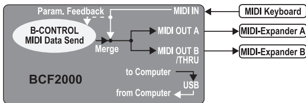
Bild 4.6: Routing och användning i Stand Alone-Mode 1
