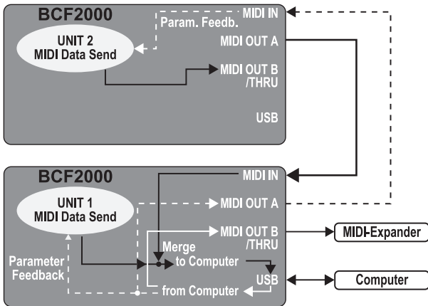
Bild 4.5: Routing i USB-Mode 4
