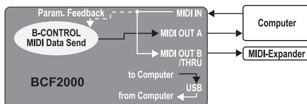
Bild 4.9: Routing och användning i Stand Alone-mode 4
