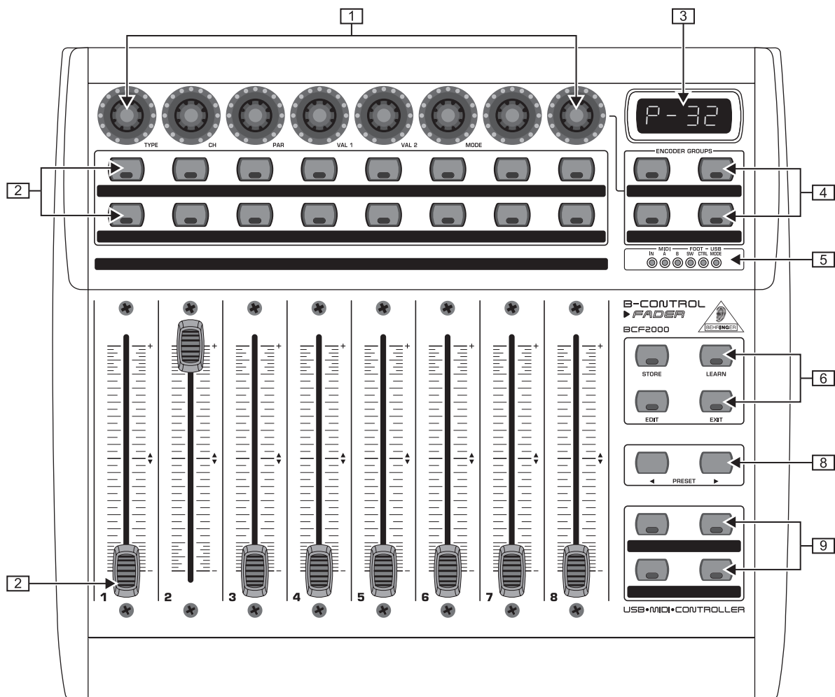
Bild 3.1: Kontrollema på B-CONTROLS ovansida
