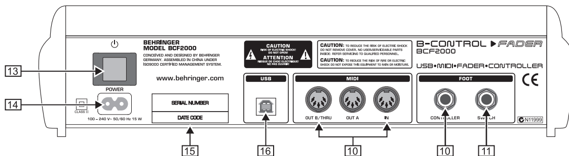
Bild 3.2: Baksidan på B-CONTROL
