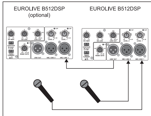
Rys. 3.1: Podłączenie mikrofonów
