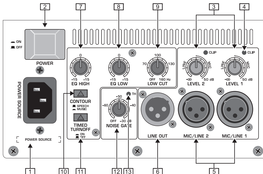
Rys. 2.1: Pola obsługi i przyłączy na stronie tylnej
