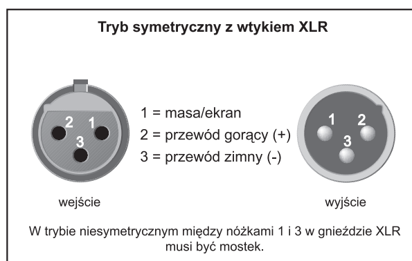
Rys. 4.1: Wtyk XLR
