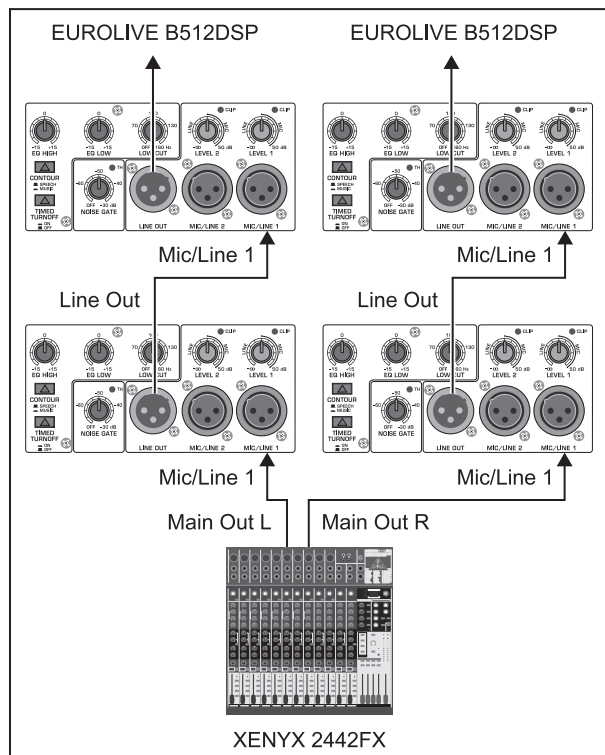
Rys. 3.3: Łączenie kilku B512DSP
