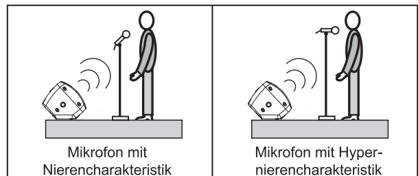
Abb. 3.3: B412DSP als Monitorlautsprecher
