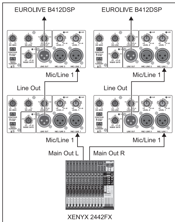
Abb. 4.3: Verkettung mehrerer B412DSP
