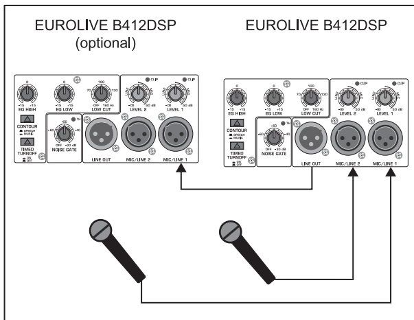
Abb. 4.1: Anschluss von Mikrofonen
