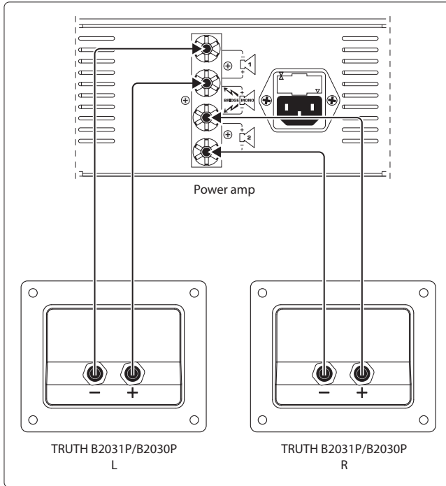
Fig. 3.1: Liitäntä vahvistimeen
